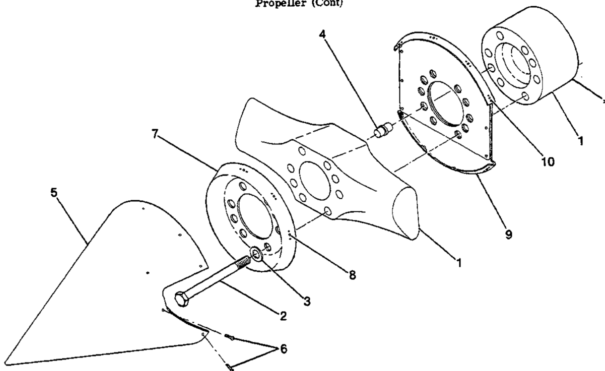
Propeller (Cont)
