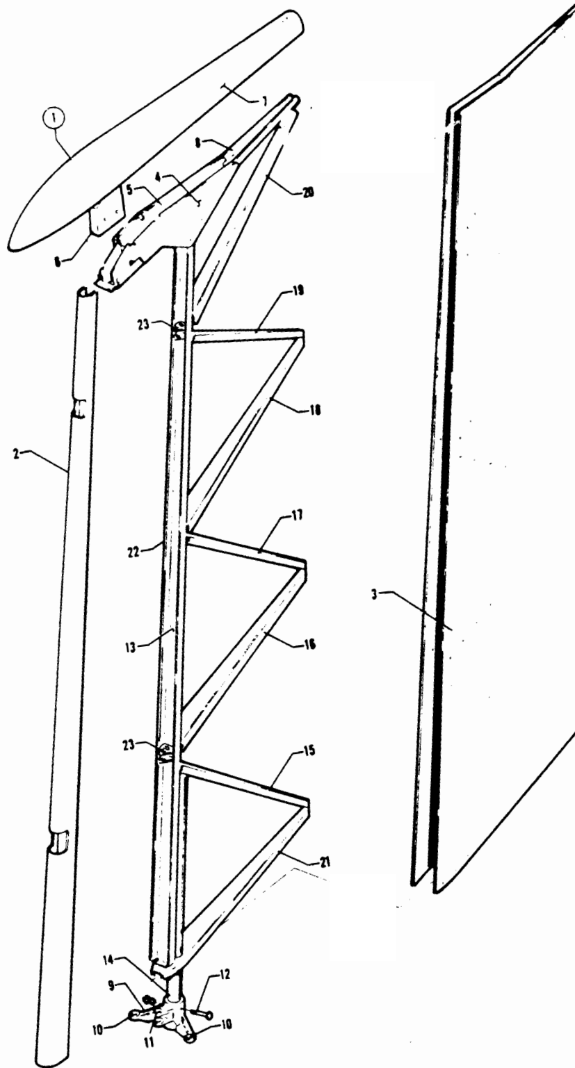
Figure 23E. Rudder Assembly "400"
