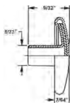
MS27980-7 Stud
